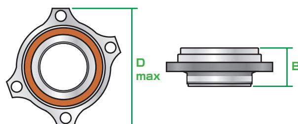
第2D世代ホイールベアリング (b)
