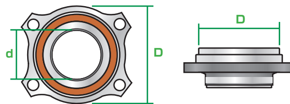
第2D世代ホイールベアリング (a)
