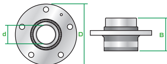
第2世代ホイールベアリング
